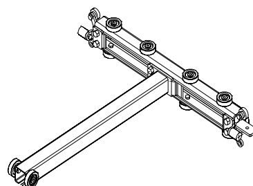
vodící vozík s unášecím ramenem
